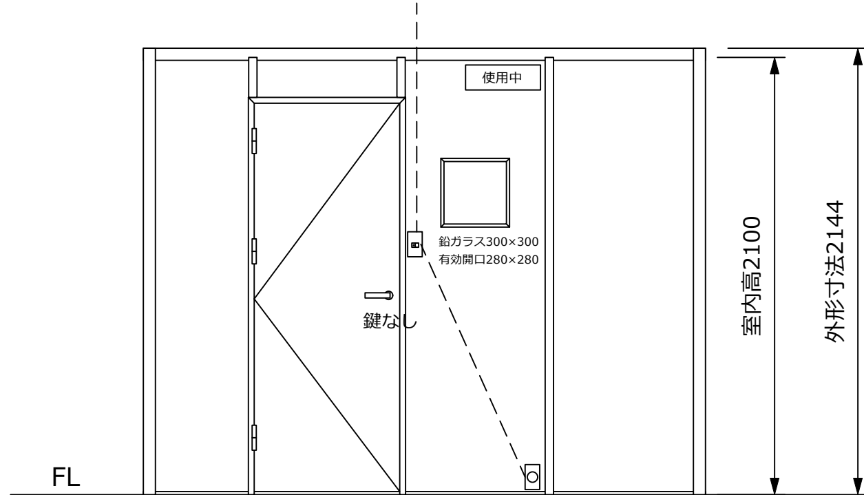
外観正面図
