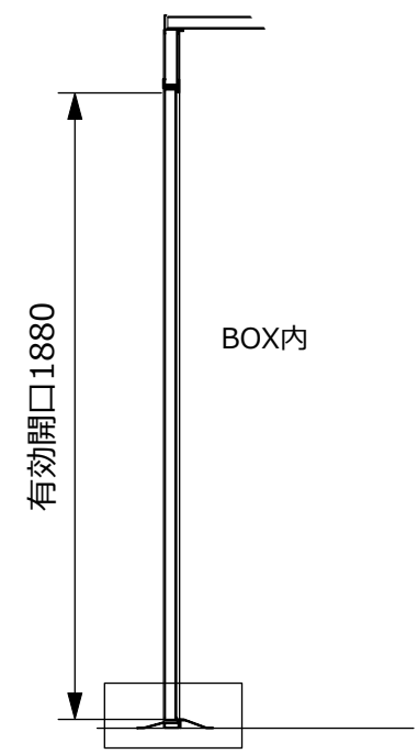
入口断面図
